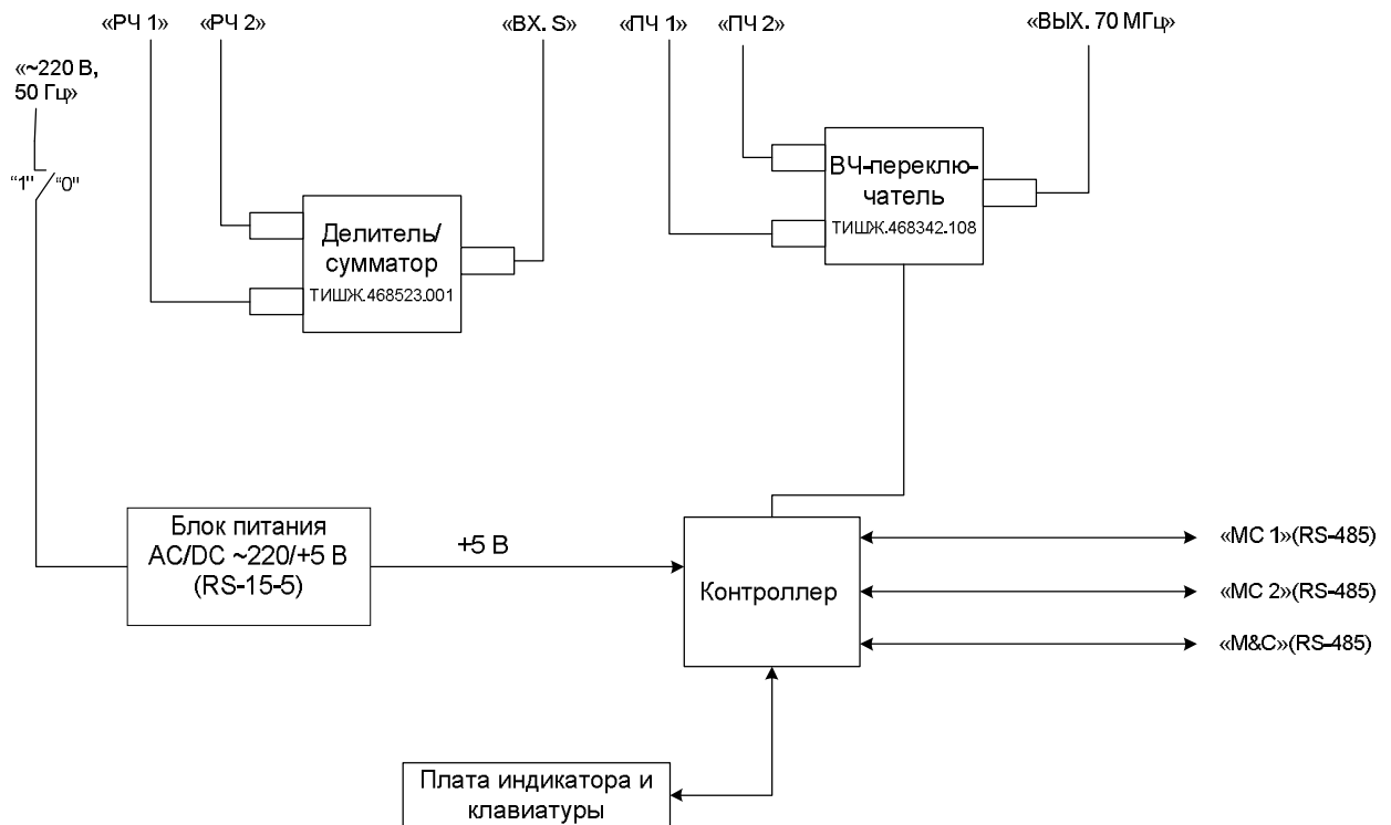
Рисунок 1.3 - Функциональная схема КРПЧ «вниз».
